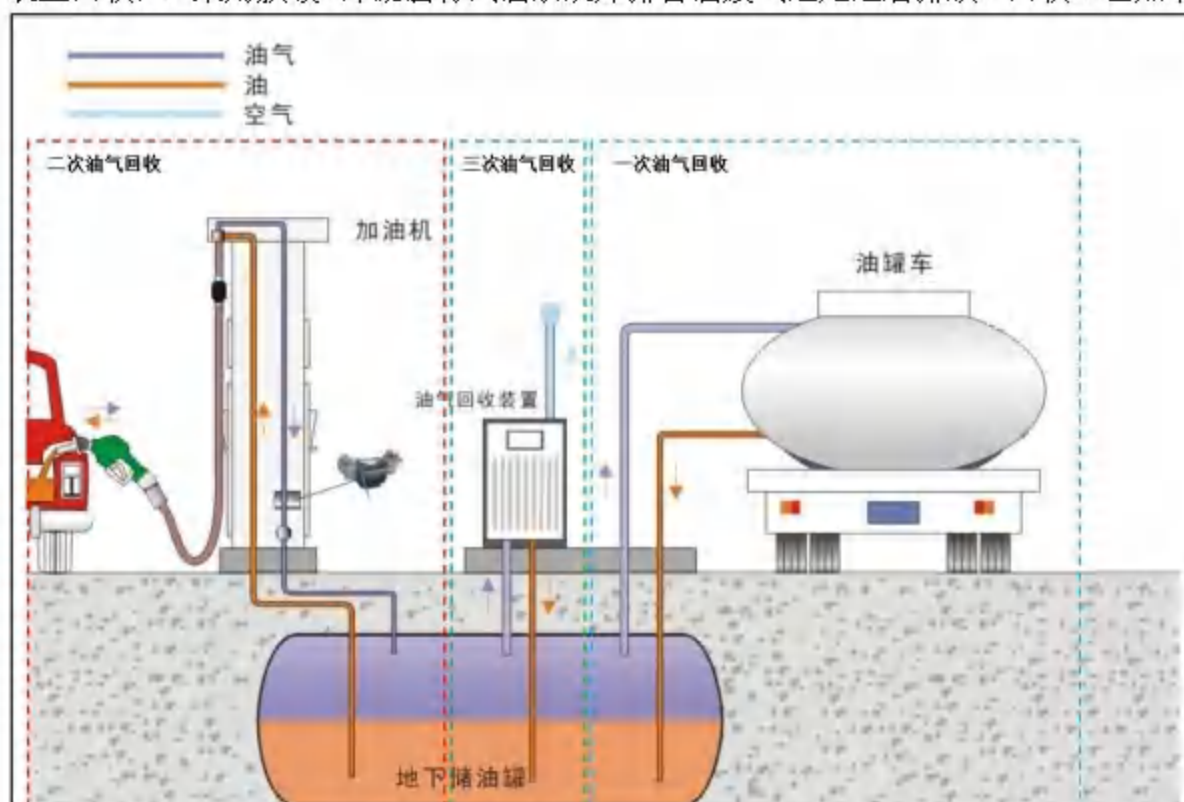
图 3-5 油气回收工艺图
