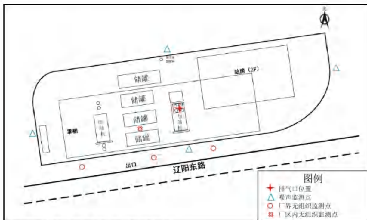
图 7-1 废气、噪声监测点位示意图
